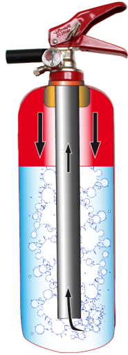
Extincteur à pression permanente
