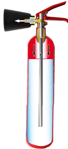
Extincteur à pression permanente
